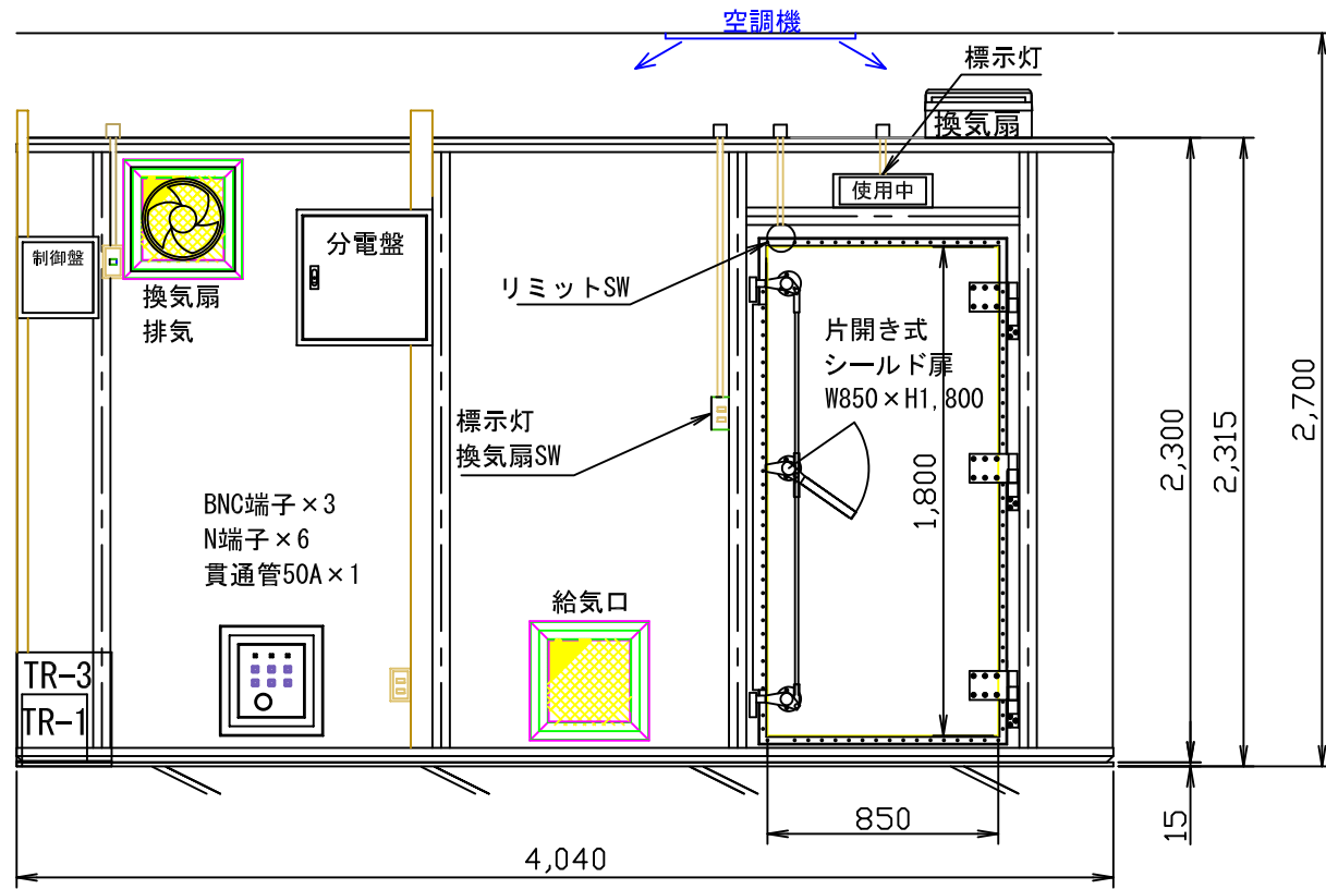
立面図 A
