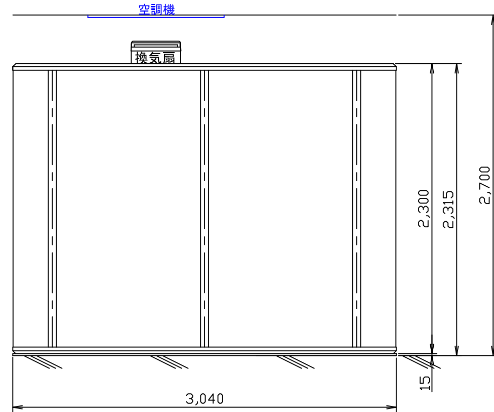
立面図 D
