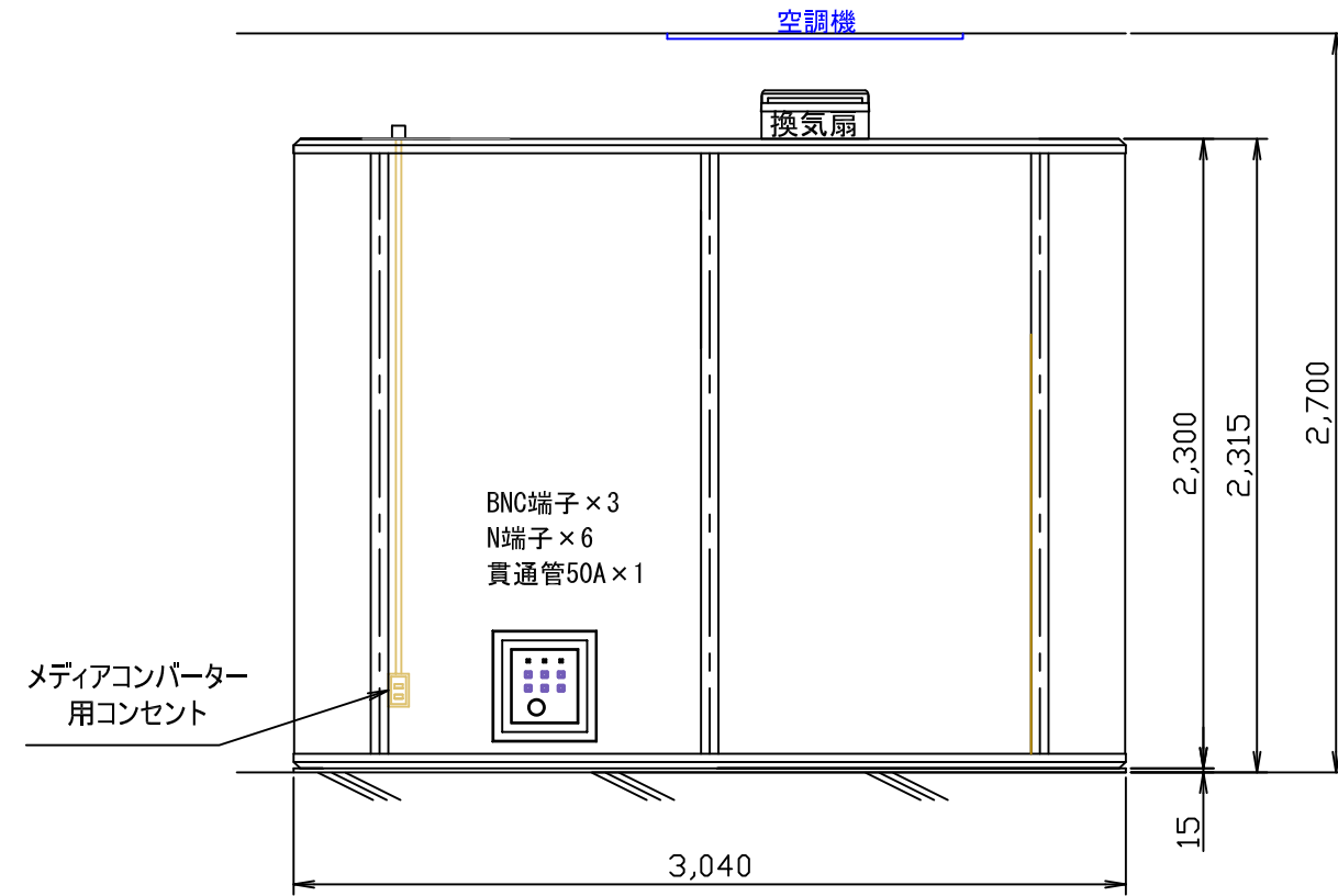
立面図 B
