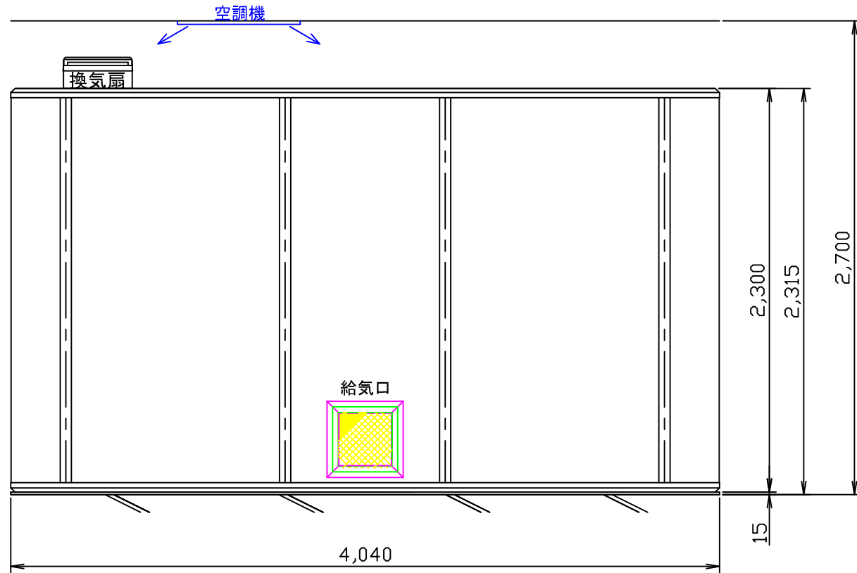
立面図 C
